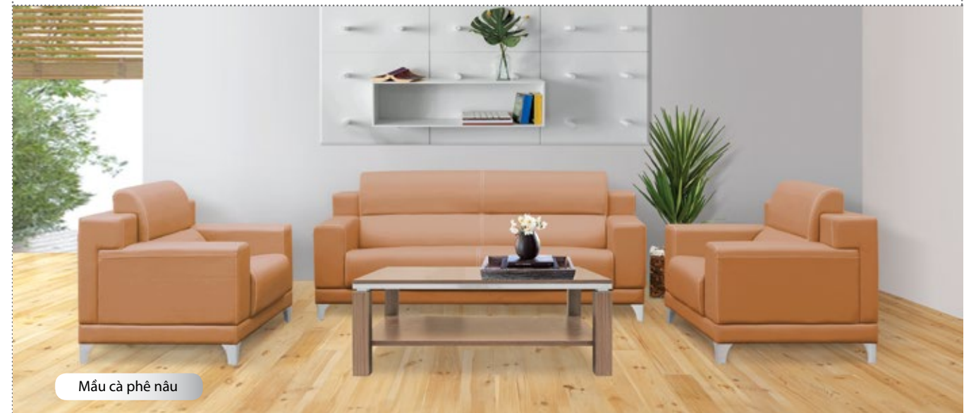
■ SP04 Băng dài: W1950xD900xH850mm - Ghế đơn: W980xD900xH850mm ■ Bàn BSP03: W1200xD600xH450
